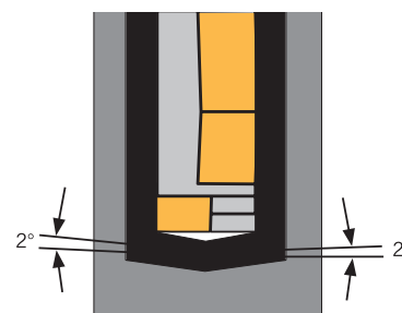
Grund ist nicht eben (2°)! Bottom is not flat (2°)! La base non è piana (2°)!
